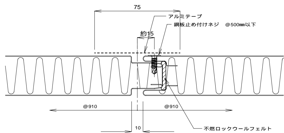
A部詳細 1/2
