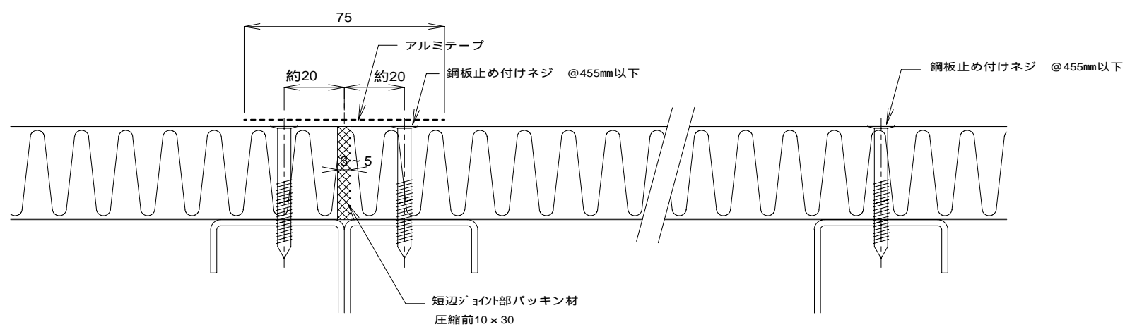
B部詳細 1/2
