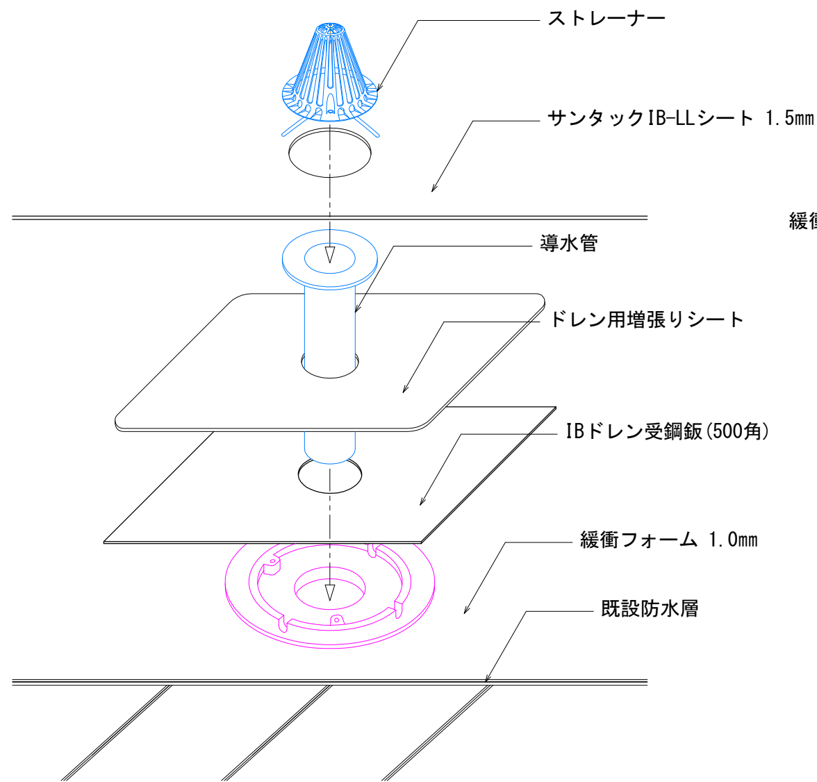
ドレン納まり斜視図 S=1:8
